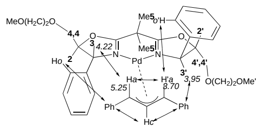
syn/syn-11e
