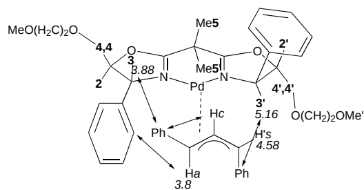
syn/anti-11e
